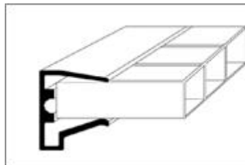
Alu-Tropfkantenprofil
