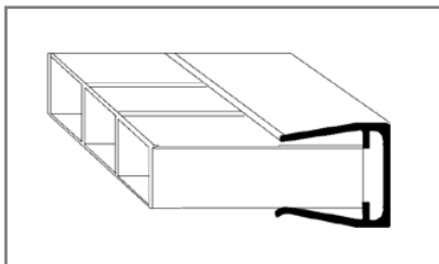
Alu-Abschlussprofil
